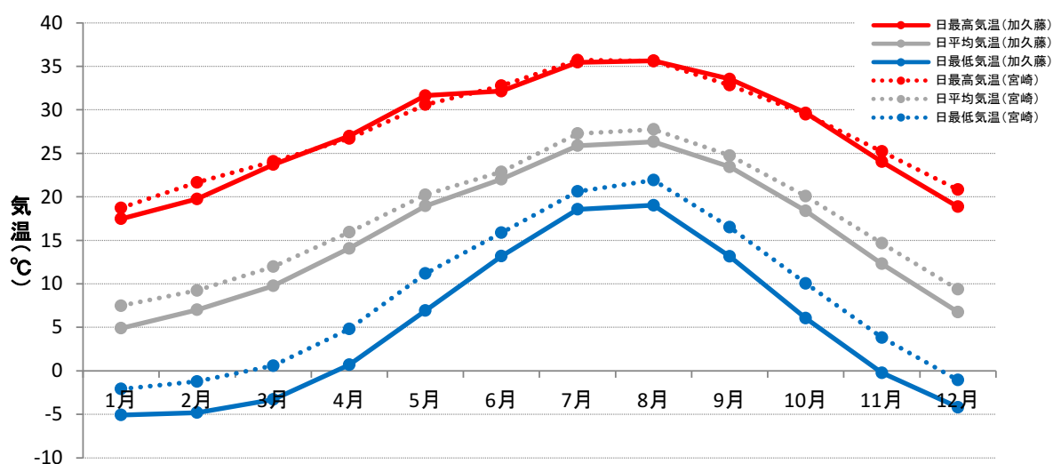
図 2.3 えびの市及び宮崎市の月別日最高・最低・平均気温 (観測所：加久藤、宮崎)
